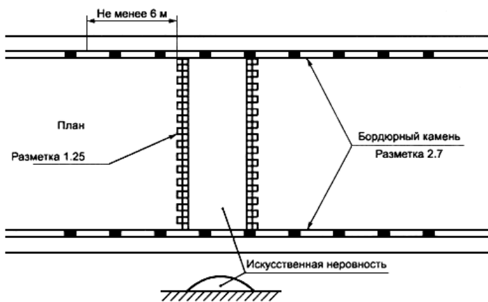
Рисунок 4 - Пример нанесения разметки 1.25 и 2.7 при устройстве ИН
