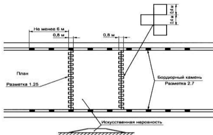
а - монолитная конструкция
