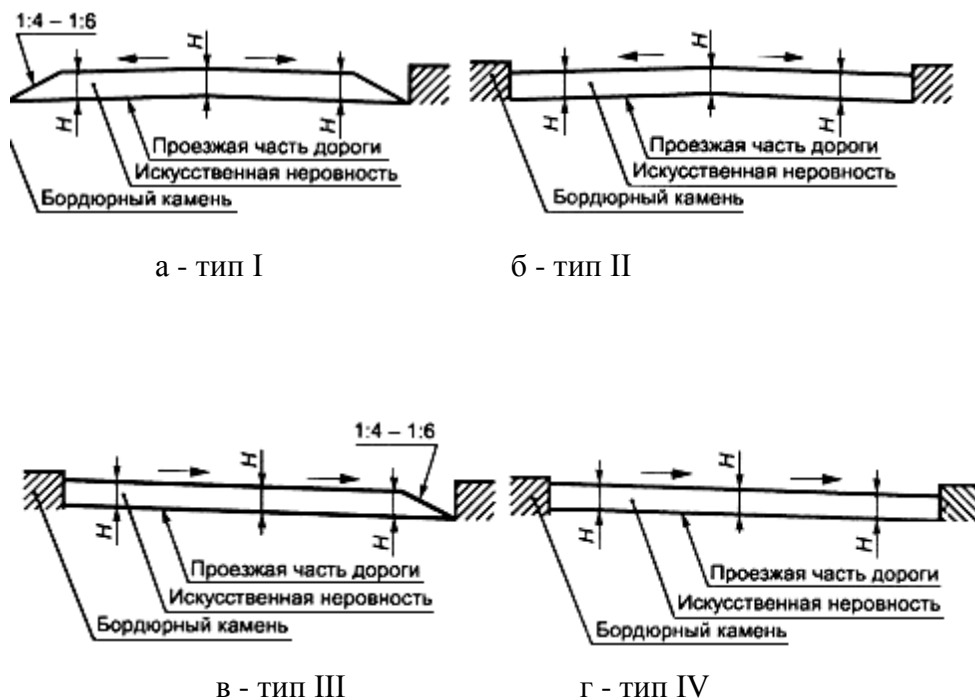
Рисунок 2 - Продольные профили ИН
